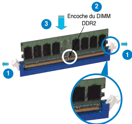
Clip de rétention déverrouillé
